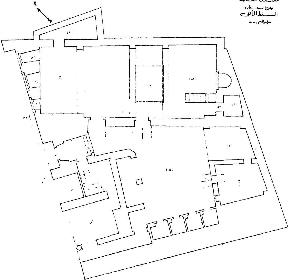
شكل ( ١ ) يبين مسقط أفقى لدرسة اسبغا
